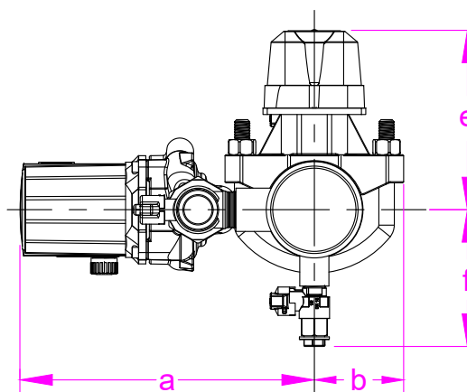
RIGHT ELEVATION
